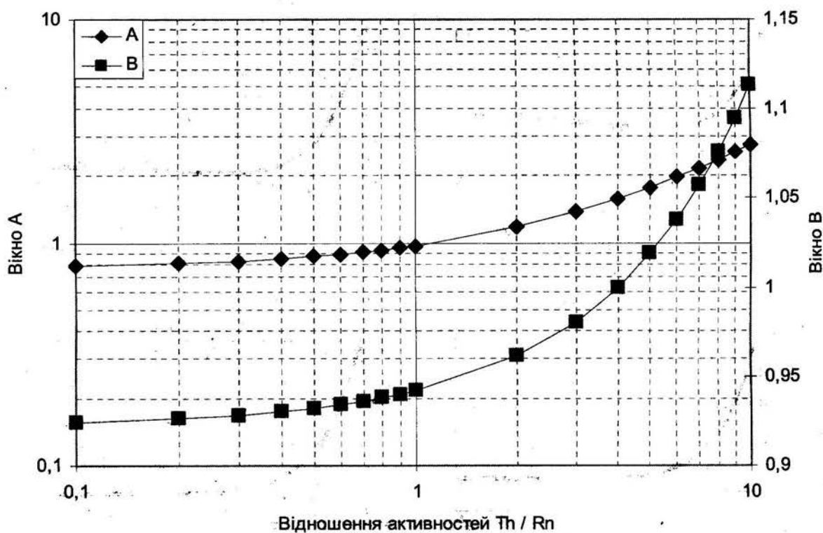
Рисунок 4. Лінійна та логарифмічна номограми співвідношень модельної середньої швидкості лічення альфа-випромінювань проби повітря ґрунту у часових інтервалах: А – 2-4 хвилини та В – 5-7 хвилини до відношення питомої активності торону ( ^{220}Rn ) та питомої активності радону ( ^{222}Rn ) за даними таблиці 1.
