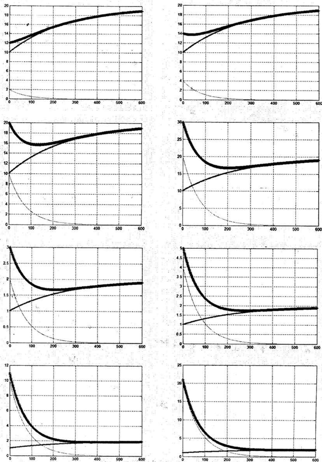
Рисунок 3. Зміна в часі (моделювання перших 10 хвилин) альфа-активності повітря за рахунок ^{222}\text{Rn} , ^{220}\text{Rn} та їх суми (жирна лінія). Залежності розглянуті для різного співвідношення компонент ^{220}\text{Rn}/^{222}\text{Rn} : 0,1; 0,2; 0,5; 1,0; 1,0; 2,0; 5,0; 10,0 (зліва направо та зверху вниз).
